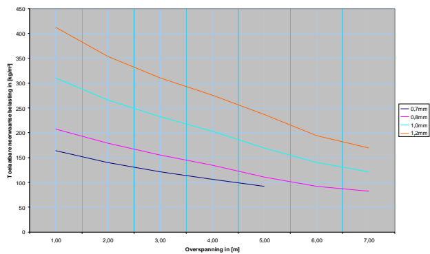
Toelaatbare neerwaartse belasting voor felsbaan 400x65 bij 2-veldoverspanning
